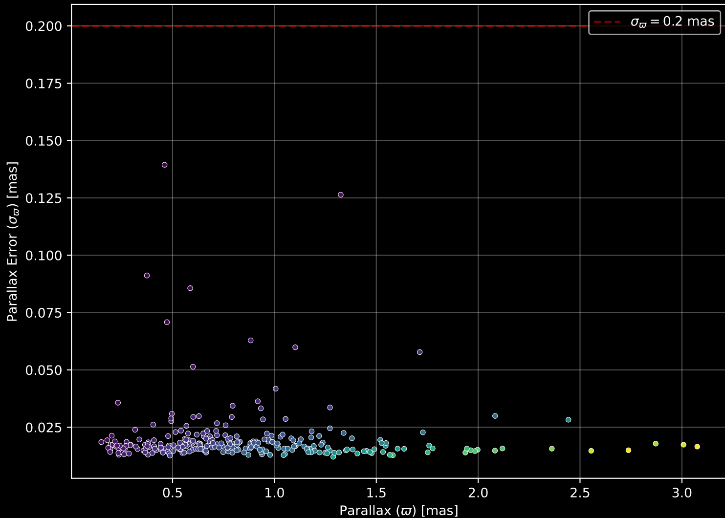
GALAH DR4 Field: [9397] Parallax Quality (n= 263)
