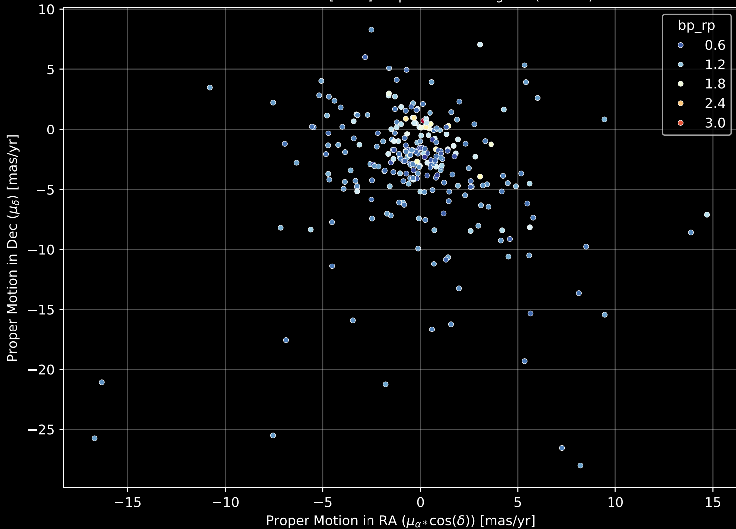
GALAH DR4 Field: [9397] Proper Motion Diagram (n= 263)
