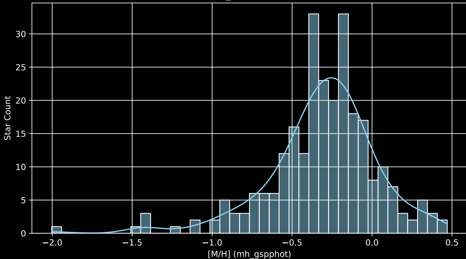
GALAH DR4 Field: [9397] [M/H] (mh_gspphot) (n= 263)
