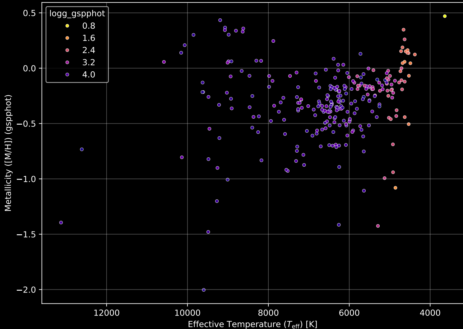
GALAH DR4 Field: [9397] Stellar Population Parameters (n = 263)
