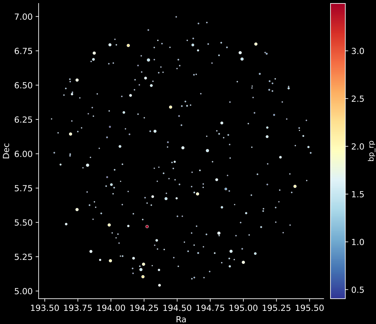
GALAH DR4 Field: [9397] Stars: 263
